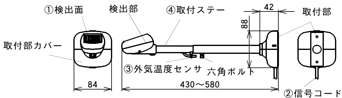
図1 センサ部
