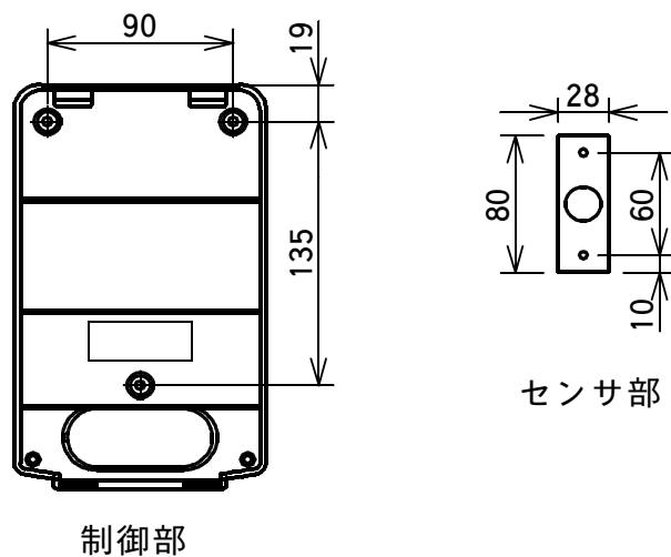
図3 取付寸法
