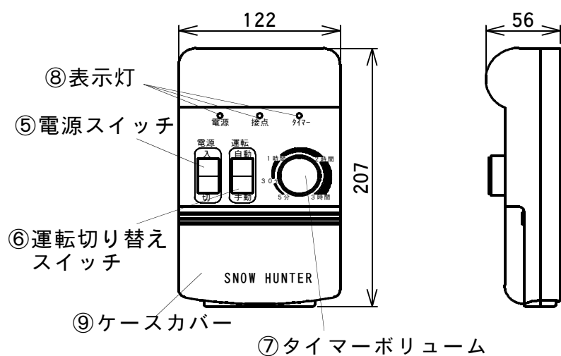
図2 制御部
