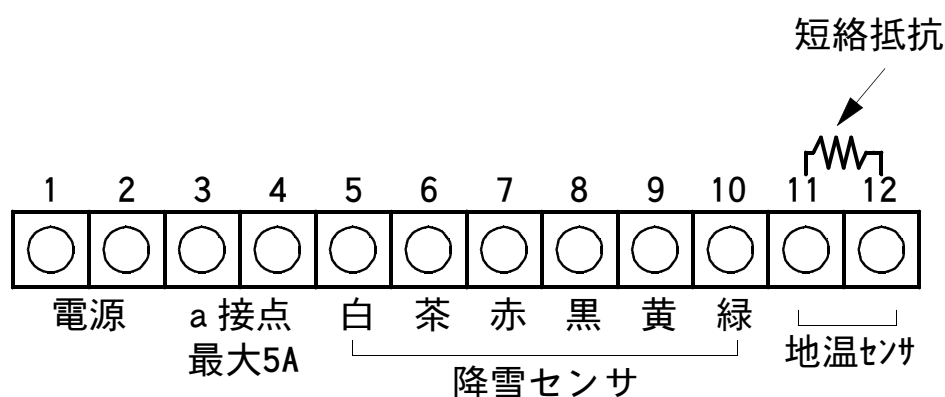
図 端子台
